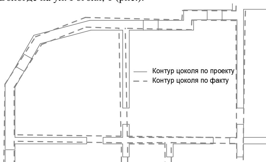
Рис. Исполнительная схема цоколя
