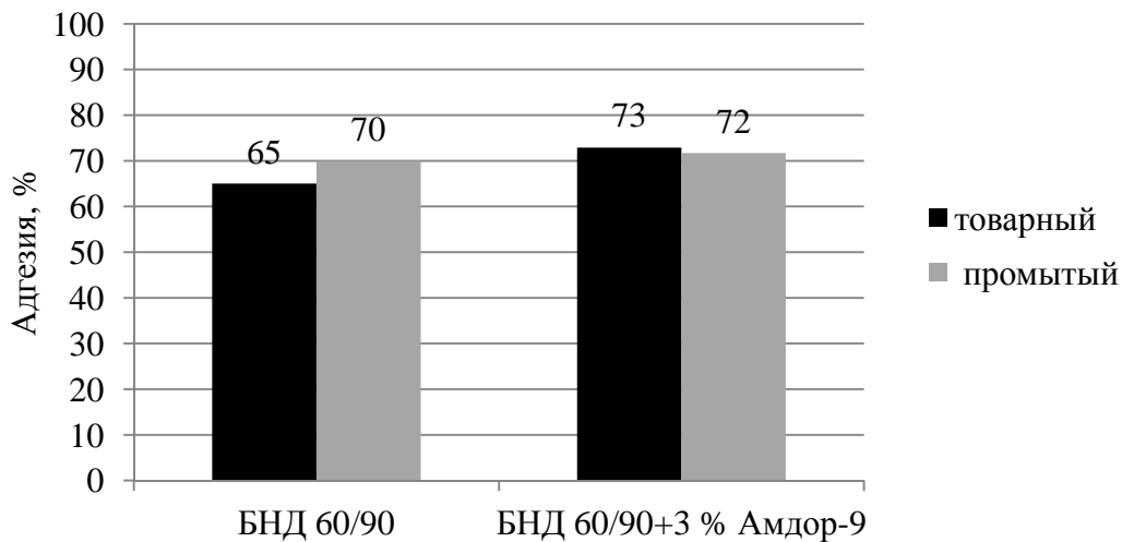
Рис. 2. Результаты определения адгезии битумных вяжущих к щебню из габбро-диабазы
