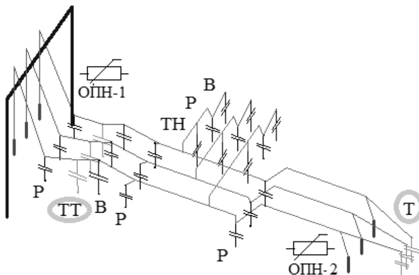
Рис. 1. Расчетная модель
