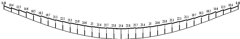
Рис. 2. Эпюра продольной силы в средней балке
