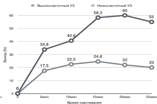
Рис. 2. Выход продукта (сточные воды) и остаточное содержание \text{CuSO}_4 (%)
