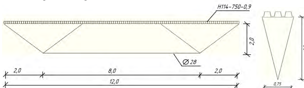
Рис. 2. Геометрические размеры плиты покрытия длиной 12 м (1 вариант)
