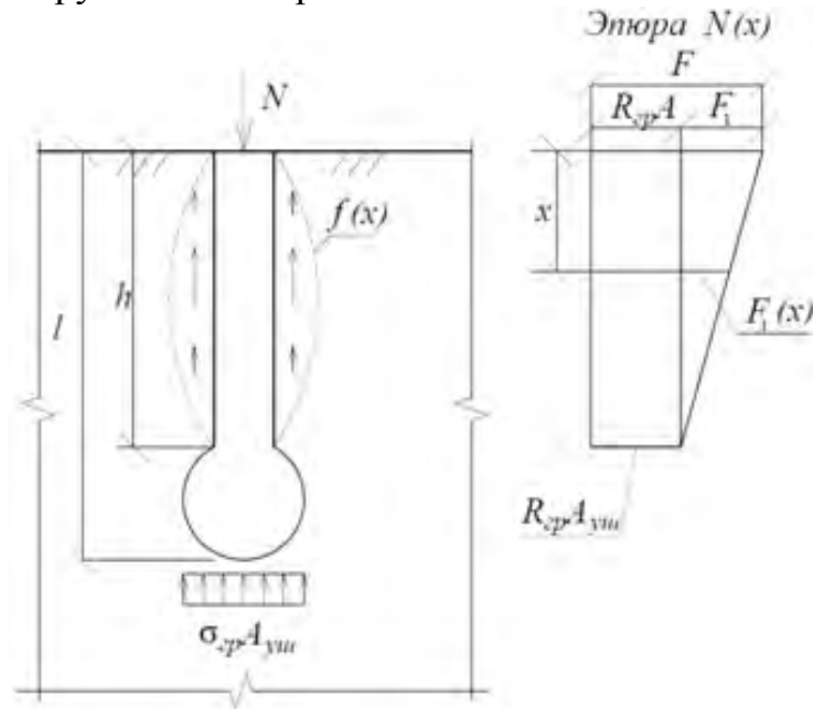
Рис. Расчетная схема сваи и эпюра N(x) от \sigma_{зр}A и f(x)
