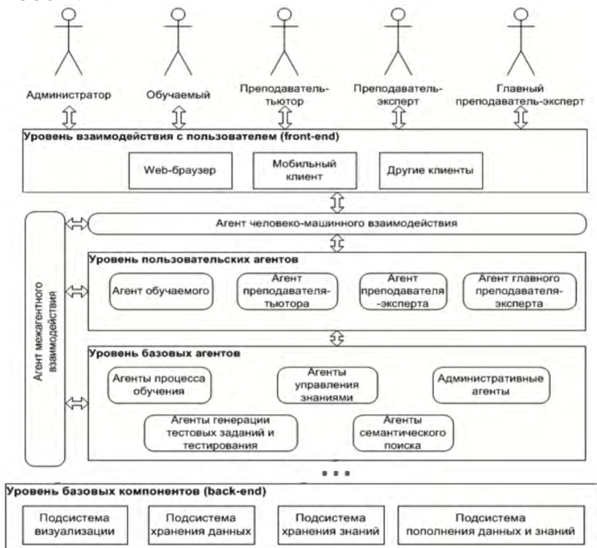
Рис. Архитектура интеллектуального агентно-ориентированного учебного комплекса
