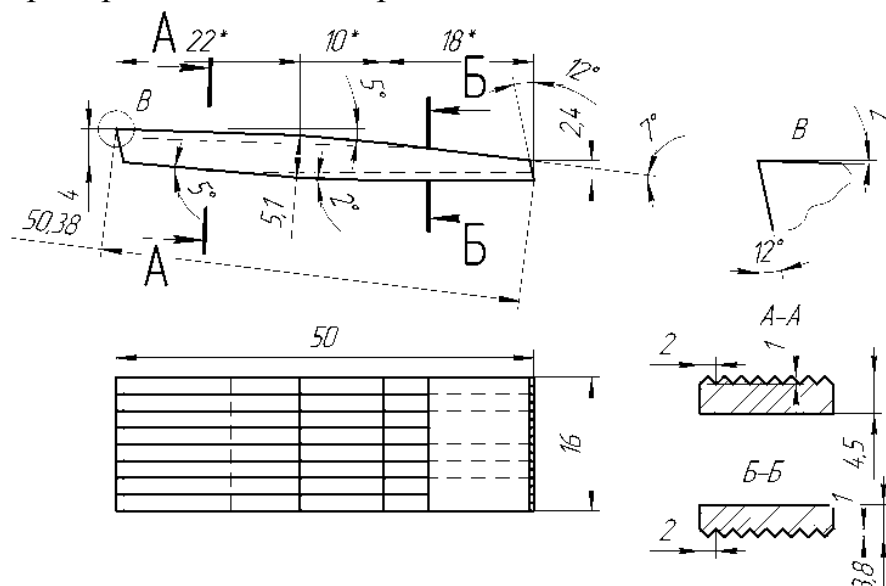
Рис. 1. Твердосплавная вставка
