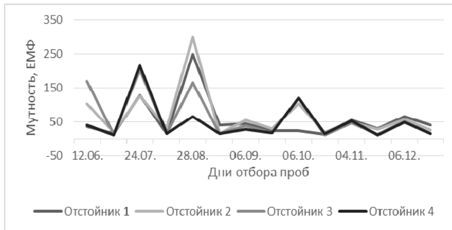
Рис. 1. Оценка эффективности работы отстойников
