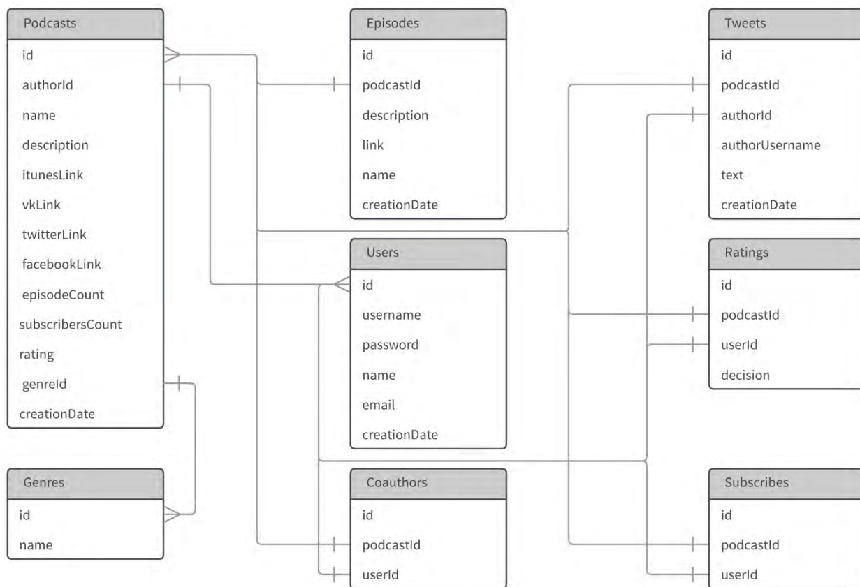
Рис. Схема базы данных
