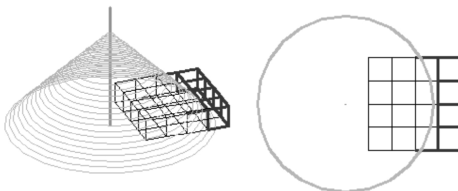
Рис. 3. Зона защиты молниеотвода и незащищенная часть здания
