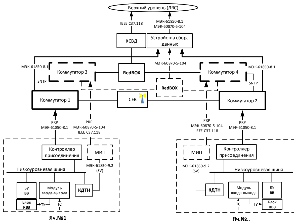
Рис. Структурная схема связи
