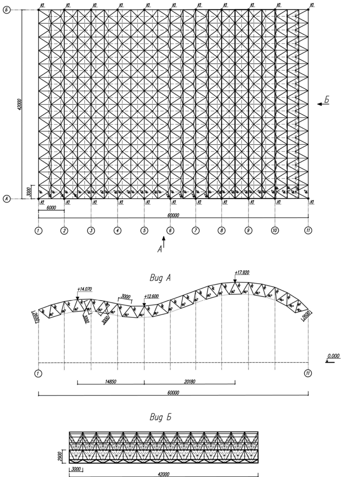
Рис. Конструкция покрытия здания теннисного корта: вид сверху, вид спереди, вид сбоку
