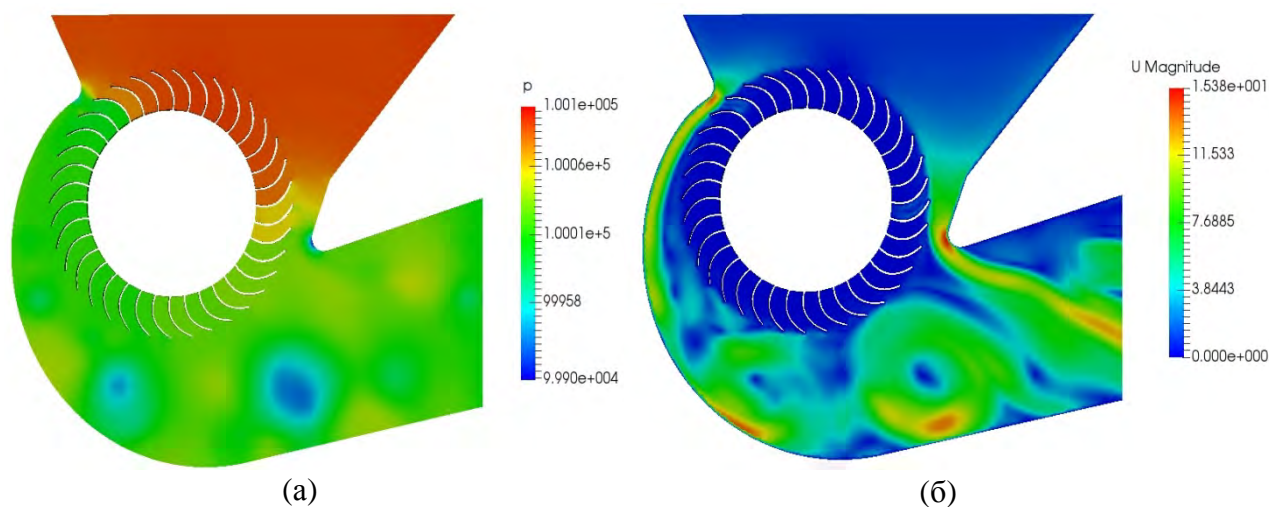
Рис. Поле давления (а) и скорости (б) в объеме ВТЗ при объемном расходе воздуха 500 \text{ м}^3/\text{ч}
