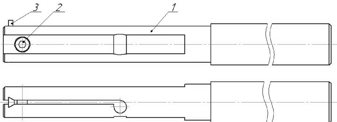
Рис. 1. Эскиз инструмента: 1 – корпус; 2 – винт; 3 – режущий элемент
