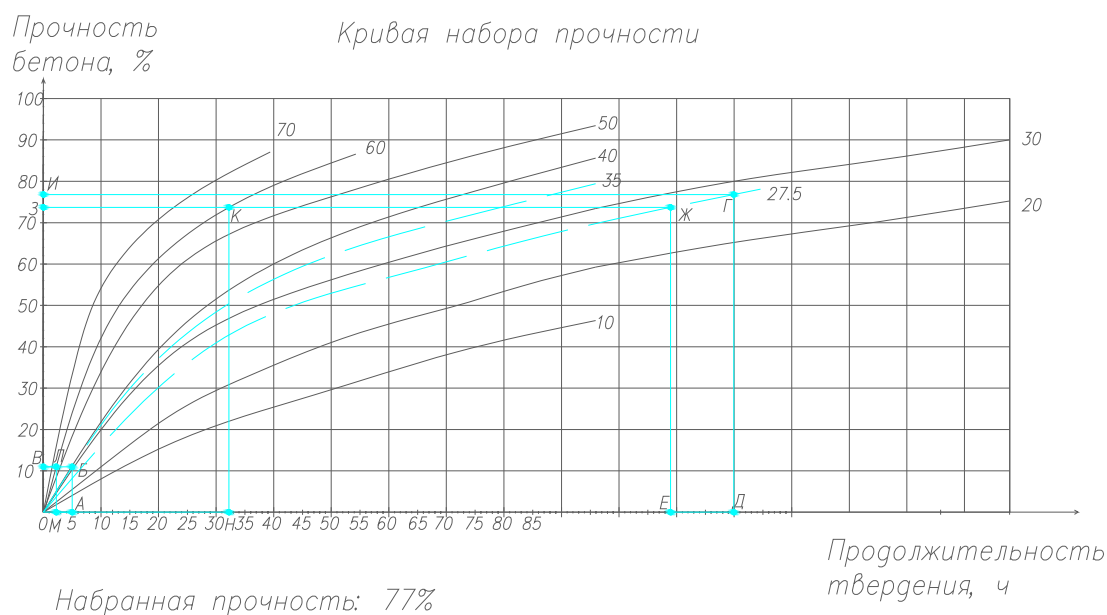
Рис. Кривая набора прочности
