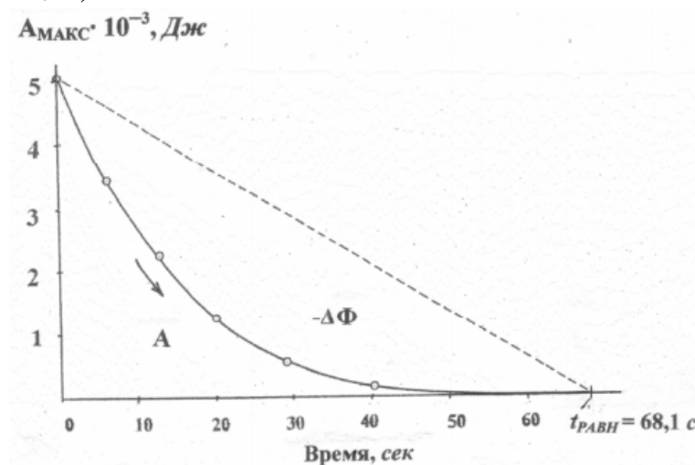
Рис. Энергетические траектории торможения маховика при равновесном и неравновесном процессах
