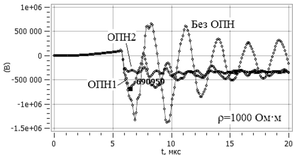
Рис. 3. Перенапряжения на силовом трансформаторе
