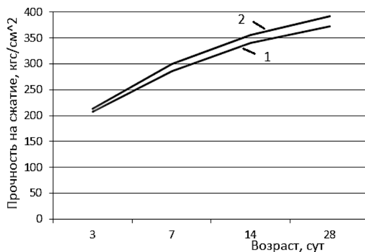
Рис. Зависимость прочности бетона от времени твердения и наличия добавки: 1 – без добавки; 2 – с добавкой «Sikament» в количестве 1,5%
