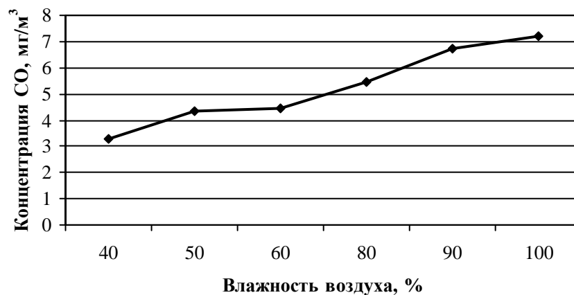
Рис. 2. Зависимость концентрации угарного газа от влажности воздуха
