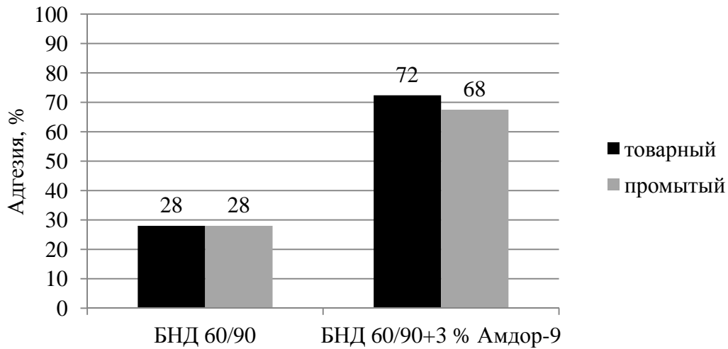
Рис. 1. Результаты определения адгезии битумных вяжущих к щебню из гранита
