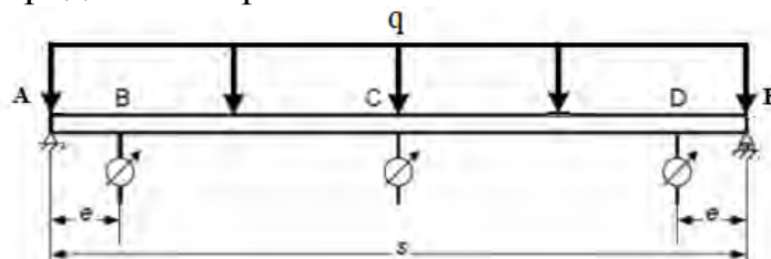
Рис. 1. Схема испытательного стенда
