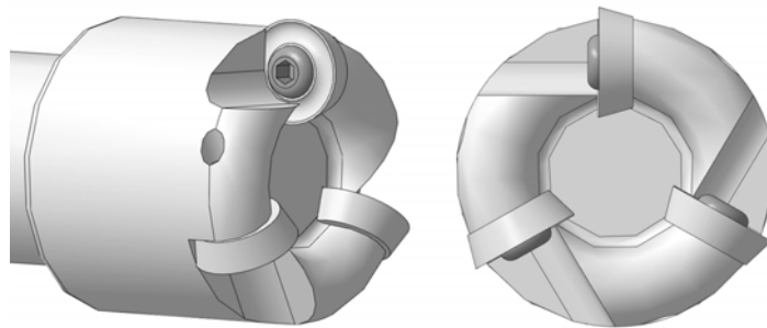
Рис. 2. 3D-модель концевой фрезы
