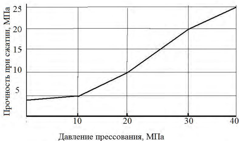
Рис. Зависимость предела прочности при сжатии от давления прессования
