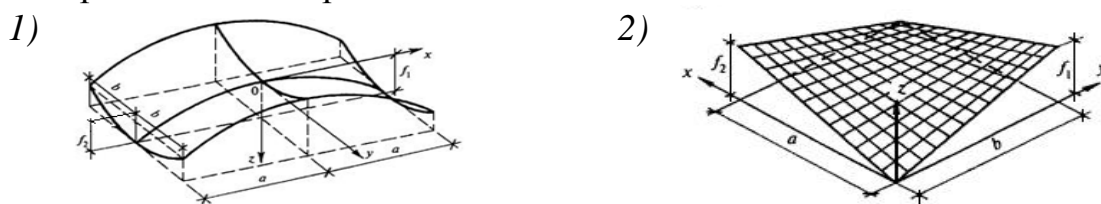
Рис. 1. Схемы оболочек с заданным центром начала координат и с направлением осей: 1) гиперболический параболоид; 2) однолепестковый гипар
