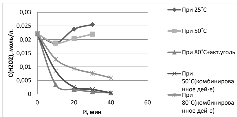
Рис. Влияние условий (УЗО, температуры, катализатора – активированный уголь) на процесс разложения пероксида водорода
