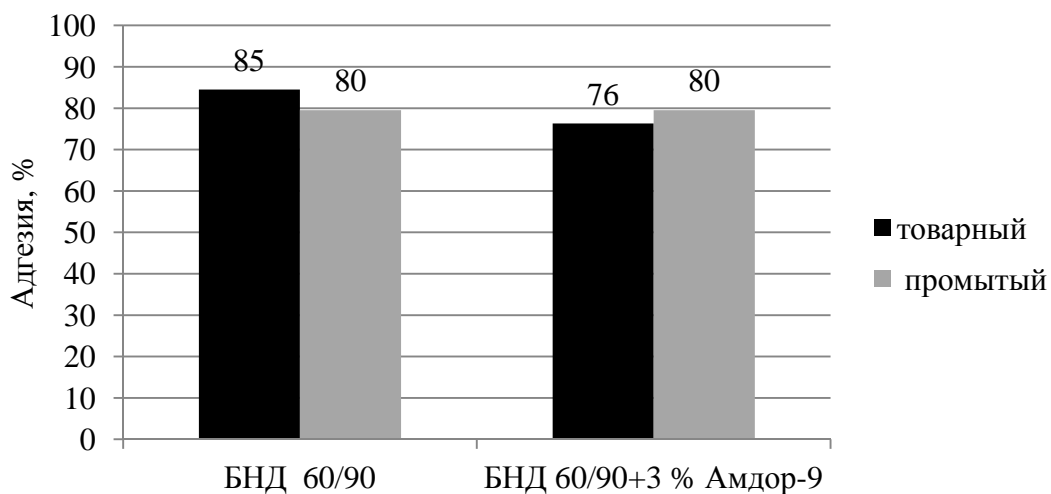
Рис. 3. Результаты определения адгезии битумных вяжущих к щебню из сталеплавильного шалка
