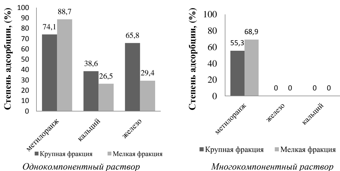
Рис. Адсорбционная способность торфа
