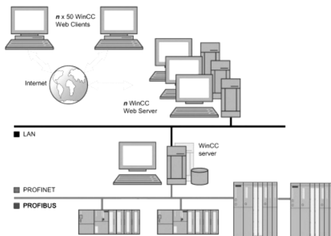
Рис. Уровни системы технологической автоматизации
