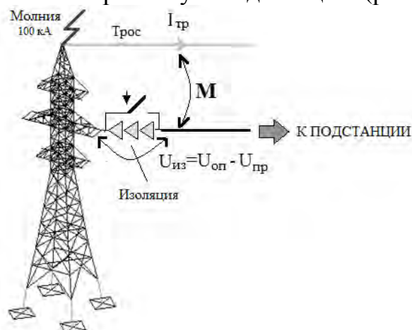
Рис. 1. Модель опоры ВЛ при ударе молнии
