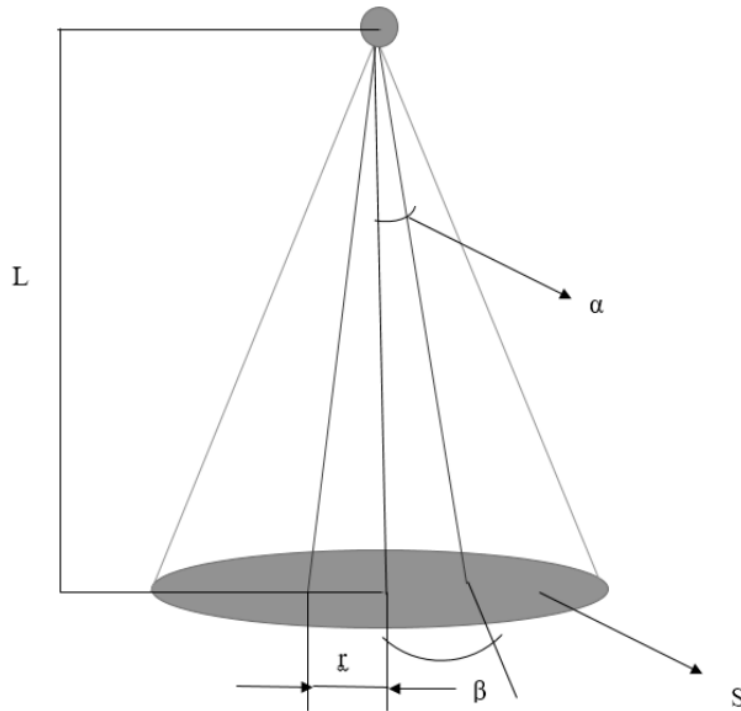
Рис. Схема распространения струи огнетушащего вещества, истекающей из оросителя автоматической установки пожаротушения
