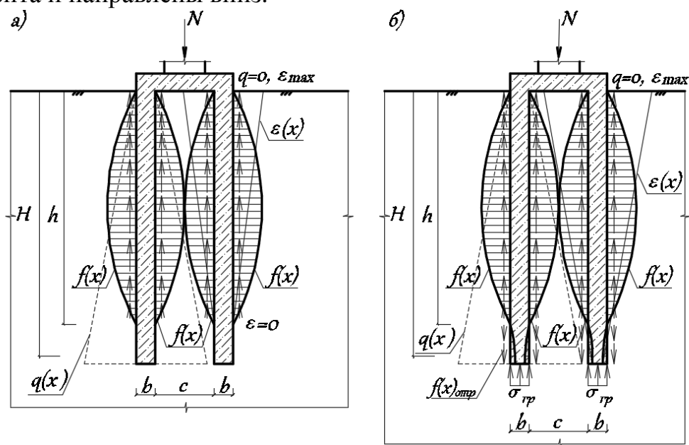
Рис. Расчетная схема двухщелевого фундамента в новой интерпретации:
