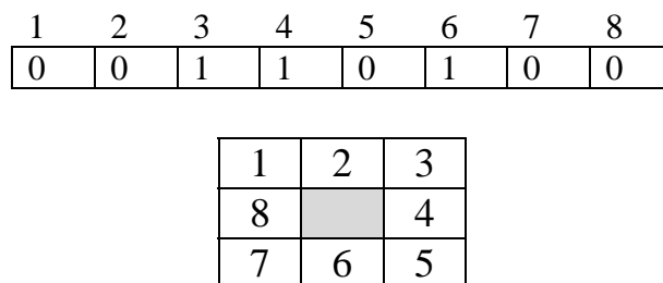
Рис. 1. Пример правила изменения состояния клетки автомата (ключа шифрования)
