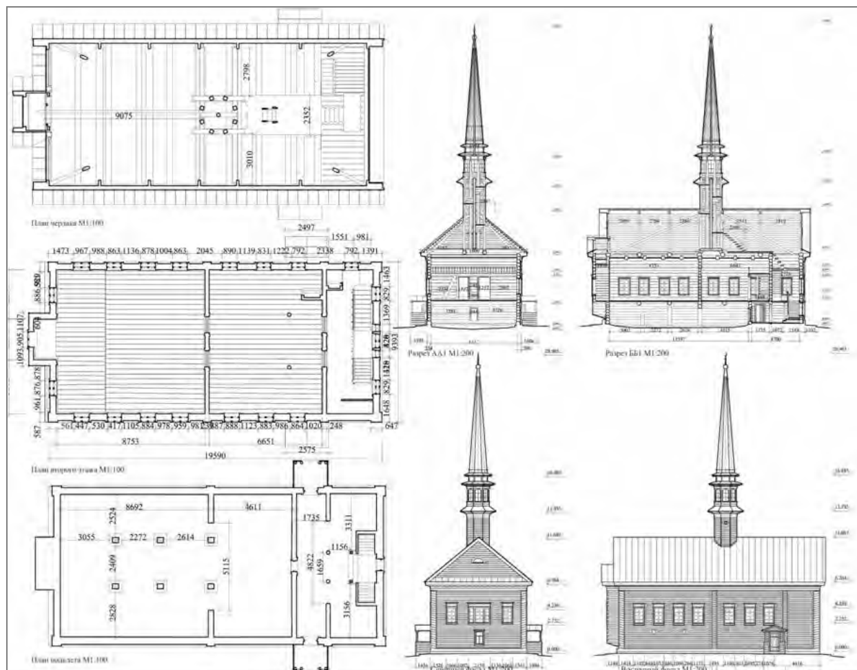
Рис. Обмерные чертежи мечети в с. Айбаш Высокогорского района Татарстана. Автор М.С. Шакуров
