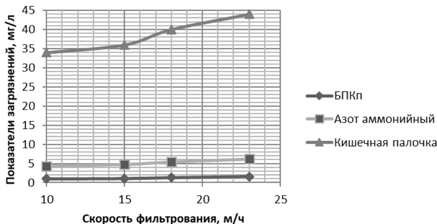
Рис. 3. Влияние скорости фильтрации на изменения показателей очистки
