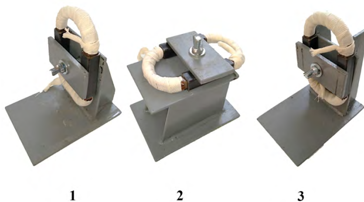
Рис. 1. Насадки для стенда: 1 – для определения остаточной прочности лобовой части обмотки; 2 – для определения усилия выдергивания статорной обмотки из паза; 3 – для определения остаточной склеиваемости витков обмотки между собой
