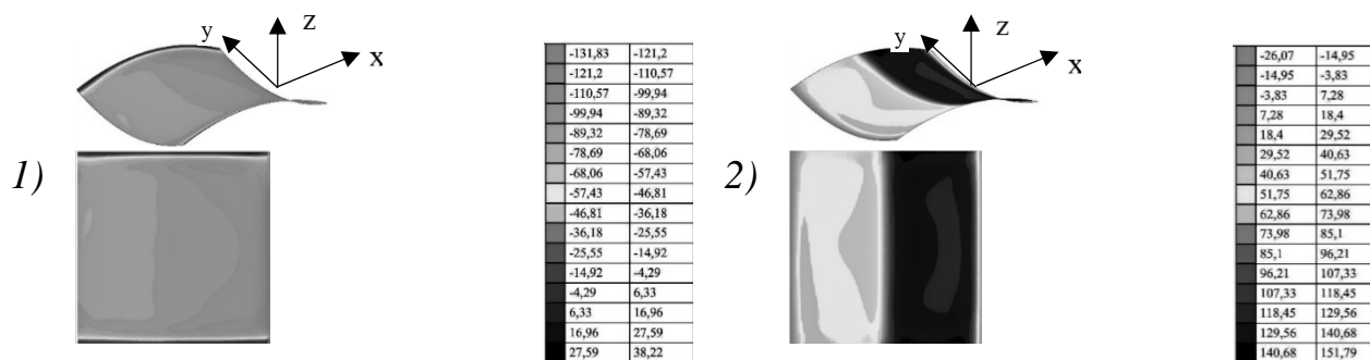
Рис. 2. Поля напряжений гиперболического параболоида с заданным центром начала координат: 1) напряжения \sigma_x ; 2) напряжения \sigma_y
