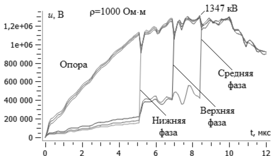
Рис. 2. Напряжение проводов ВЛ при ударе молнии с током 100 \text{ кА} в вершину опоры (рис. 1)
