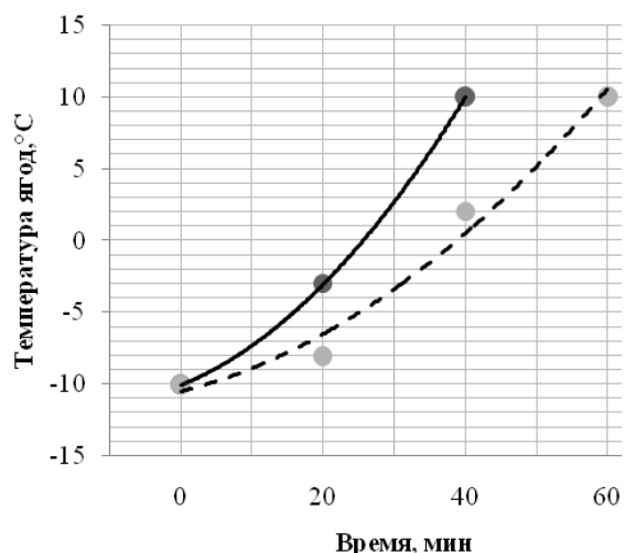
Рис. График изменения температуры замороженных ягод при их размораживании
