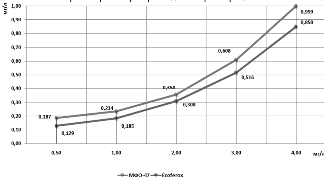
Рис. 2. Результаты эксперимента (представлены средние значения по каждой концентрации раствора)
