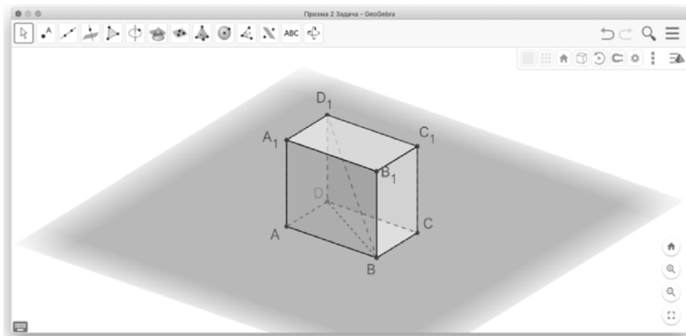
Рис. Чертеж к задаче в интерактивной геометрической среде
