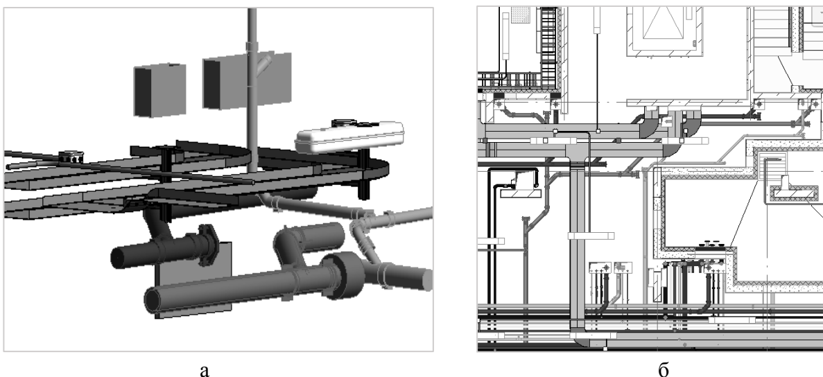
Рис. 2. Вид участка сетей в 3D и фрагмент плана техподполья с инженерными сетями
