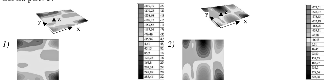
Рис. 3. Поля напряжений однолепесткового гипара с заданным центром начала координат в точке опущенного угла: 1) напряжения \sigma_x 2) напряжения \sigma_y
