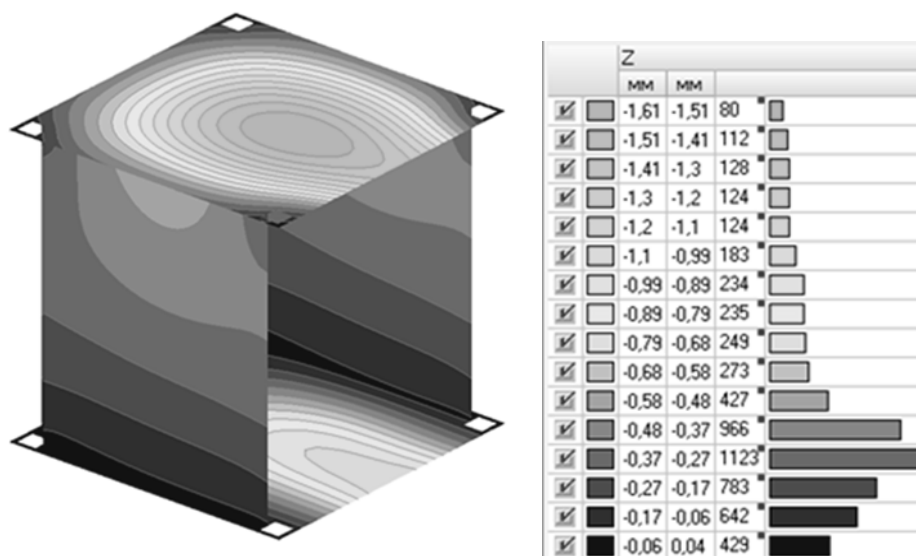
Рис. 2. Ячейка каркаса с заполнением из полнотелого кирпича с трех сторон (жесткое примыкание)
