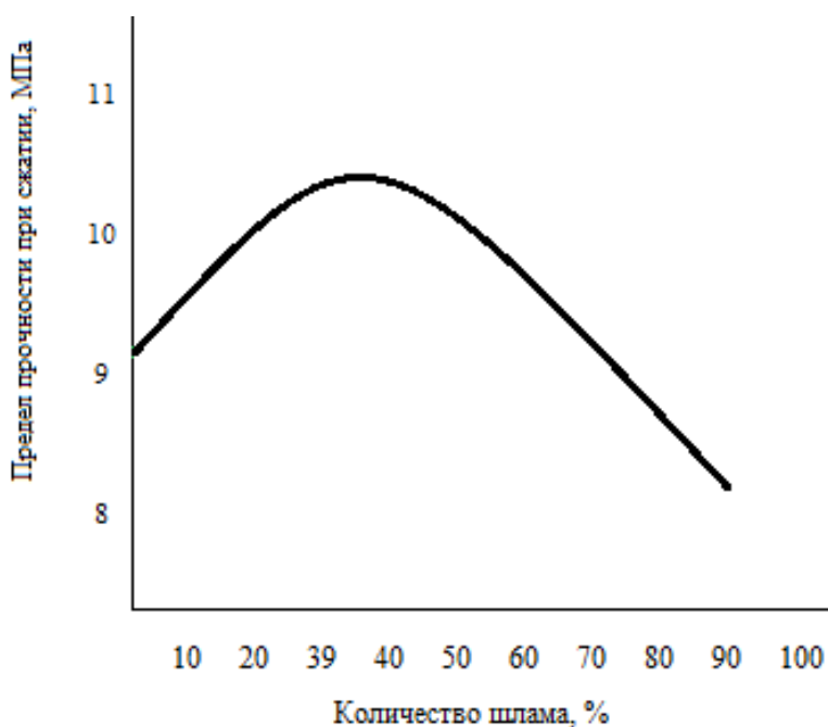
Рис. Зависимость прочности при сжатии мелкозернистого бетона от количества сухого шлака
