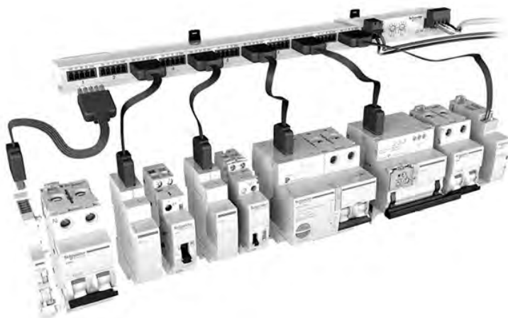
Рис. 2. Модульная аппаратура
