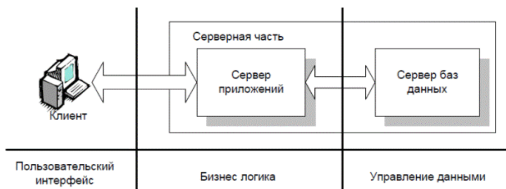
Рис. Схема архитектуры приложения
