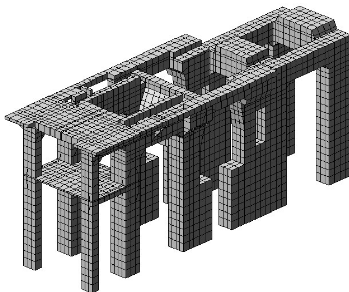
Рис. 2. Расчётная схема фундамента в программном комплексе ЛИРА-САПР2017
