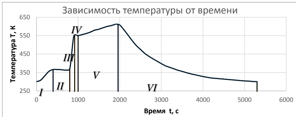
Рис. 1. График зависимости температуры нагрева образцов от времени
