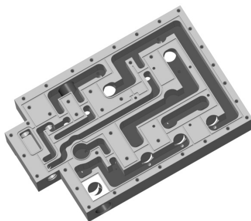
Рис. 2. Монтажная плита (вид снизу)
