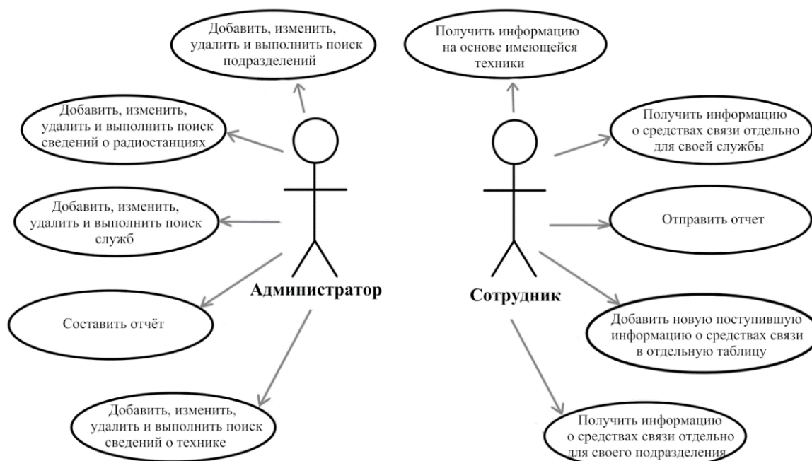
Рис. USE-CASE диаграмма
