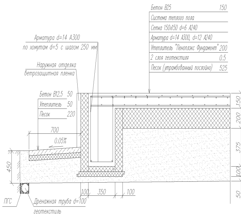
Рис. Конструкция УШП
