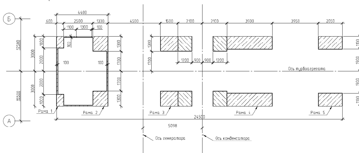
Рис. 1. План существующих конструкций фундамента на отм. 0,000
