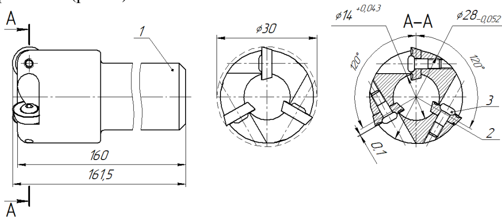
Рис. 1. Фрагмент сборочного чертежа корпуса концевой фрезы: 1) корпус фрезы; 2) твердосплавная пластинка; 3) винт-штифт
