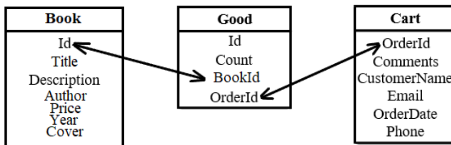
Рис. 1. Отношения между сущностями
