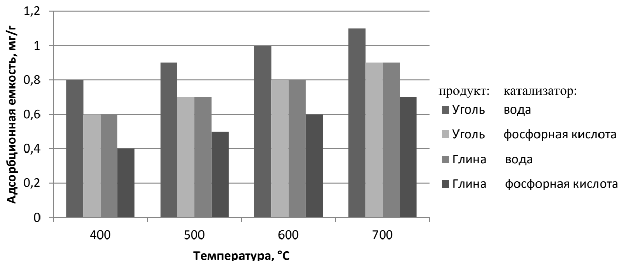
Рис. 2. Зависимость адсорбционных свойств от технологических параметров
