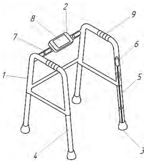
Рис. 1. Автоматически адаптируемые ходунки
