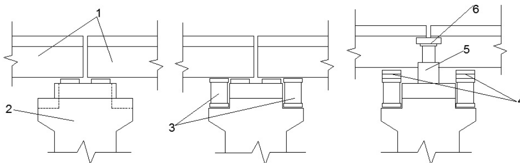
Рис. Этапы технологии поднятия пролетных строений мостов с помощью гидравлических домкратов
