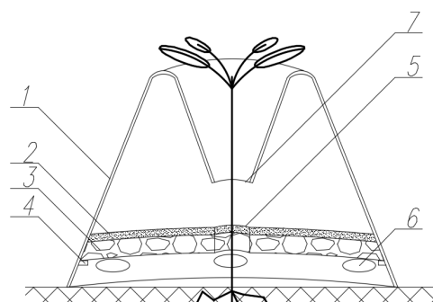
Рис. Общий вид устройства для орошения растений
