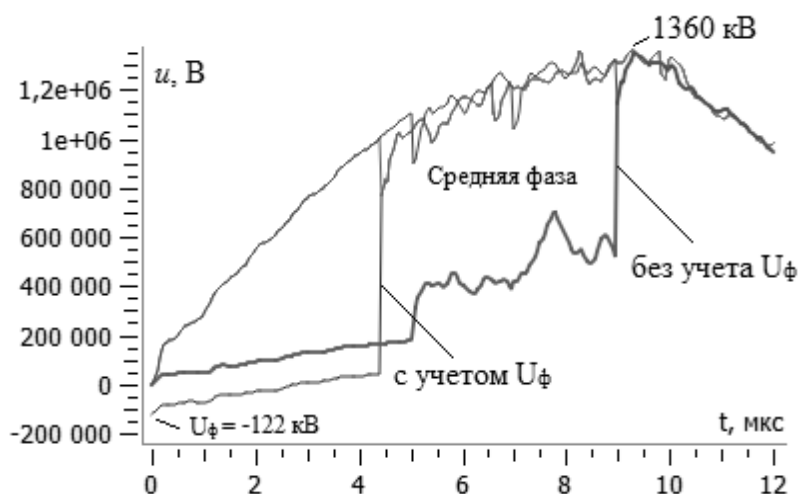
Рис. 3. Напряжение средней фазы ВЛ при ударе молнии с током 100 \text{ кА} в вершину опоры (рис. 1) с учетом и без учета рабочих напряжений
