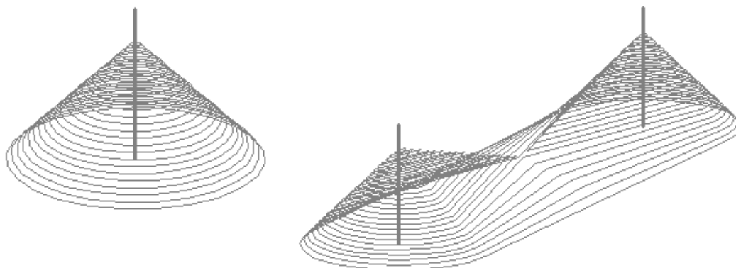
Рис. 1. Каркас зоны защиты одиночного и двойного молниеотвода
