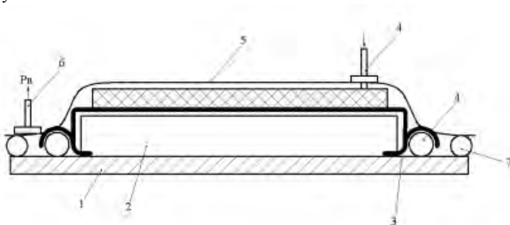
Рис. 2. Схема сборки технологического пакета для пропитки под вакуумом, где 1 – формообразующая оснастка; 2 – слой углеродной ткани арт. 3673 ф. «Porcher»; 3 – слой дренажной и жертвенной ткани; 4 – впитывающий штуцер; 5 – распределительная сетка; 6 – штуцер вакуумной линии; 7 – жгут замазка; 8 – вакуумный мешок
