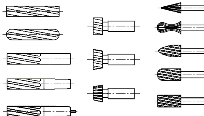
Рис. 1. Сменные концевые вставки
