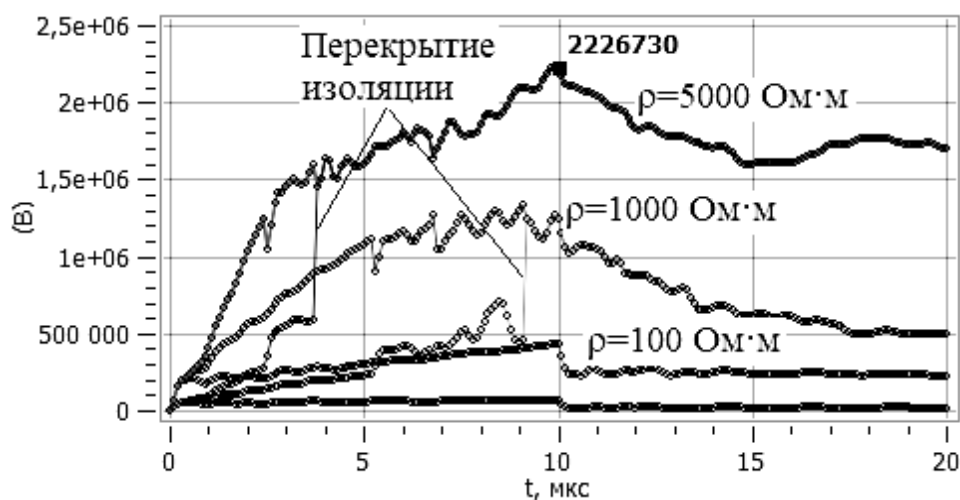
Рис. 2. Потенциалы провода и опоры при ударе молнии в опору
