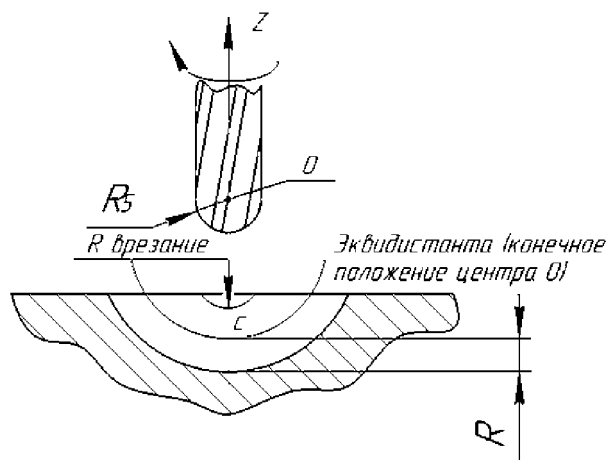
Рис. 2. Схема обработки сканированием
