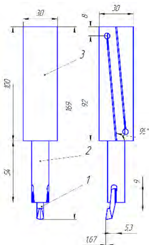
Рис. 2. Сборный долбежный резец
