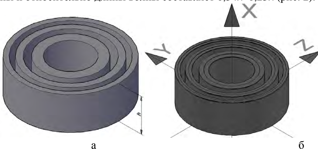
Рис. 2. Пример конструкций фазоинверторных зон из диэлектрика при: а) фокусировке на бесконечность; б) фокусировке в точку
