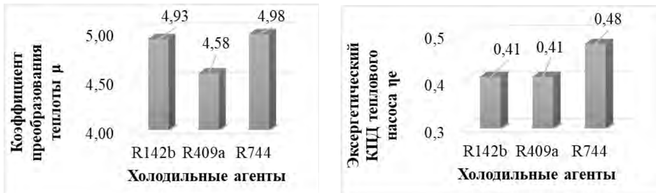
Рис. Выбор хладагента при t_0 = 10^\circ\text{C} и t_k = 60^\circ\text{C}
