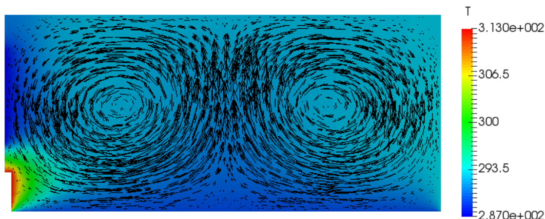
Рис. 1. Температурное поле и движение потока воздуха в комнате при использовании стационарного отопительного прибора
