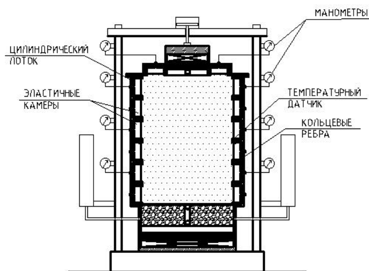
Рис. 2. Схема устройства
