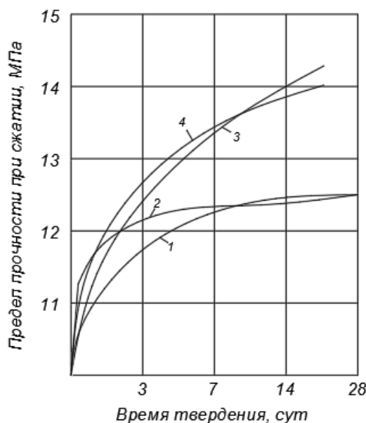
Рис. Зависимость прочности цементного камня от времени при различных технологических приемах:
