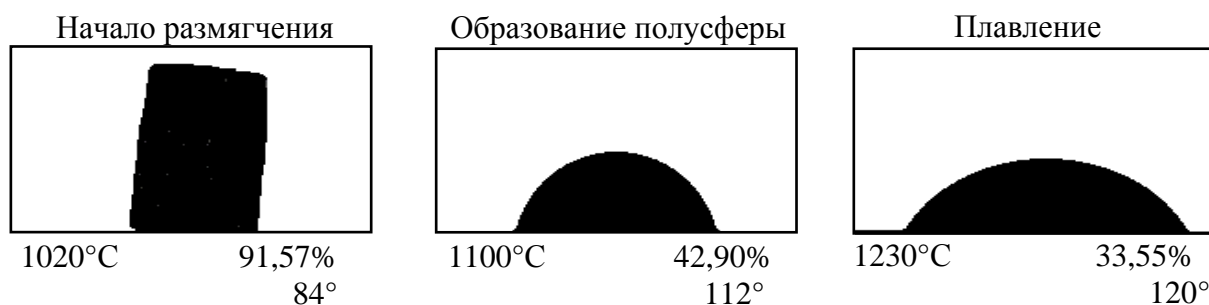
Рис. Результаты определения плавкости и краевого угла смачивания глазури оптимального состава серии 2
