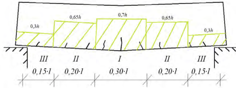
Рис. Зоны балки с предельными значениями длин трещин по [2]
