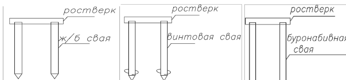
Рис. Виды свайного фундамента
