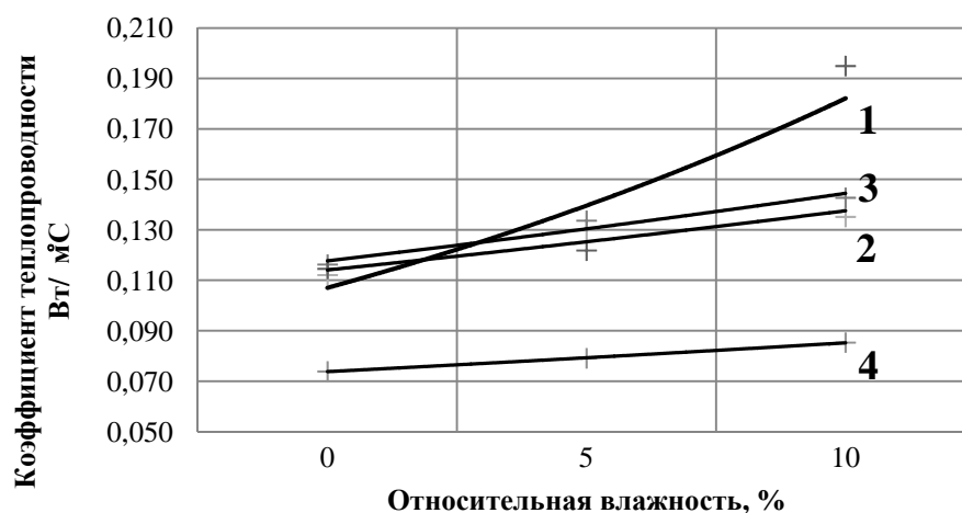
Рис. График зависимости коэффициента теплопроводности от относительной влажности опытного образца
