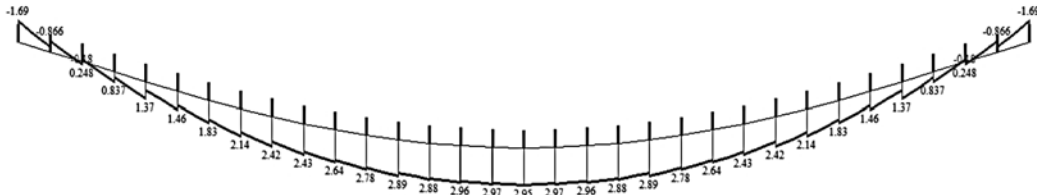
Рис. 1. Эпюра изгибающего момента в средней балке
