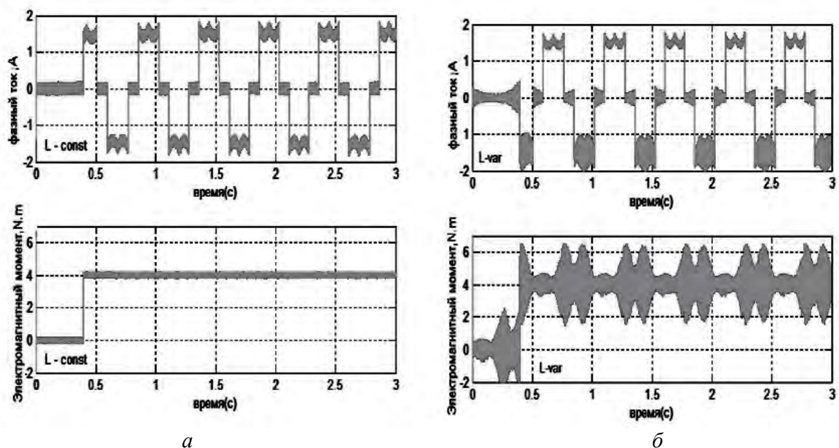
Рис. 2. Осциллограммы тока и электромагнитного момента вентильного двигателя при: а – постоянной индуктивности двигателя, б – при наличии зависимости индуктивности от угла поворота ротора двигателя
