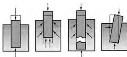
Рис. 1. Влияние морозного пучения на фундамент
