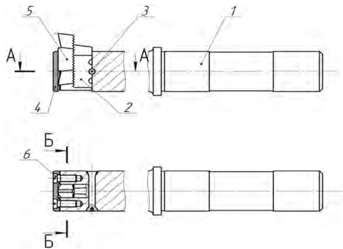
Рис. Резец долбежный переналаживаемый
