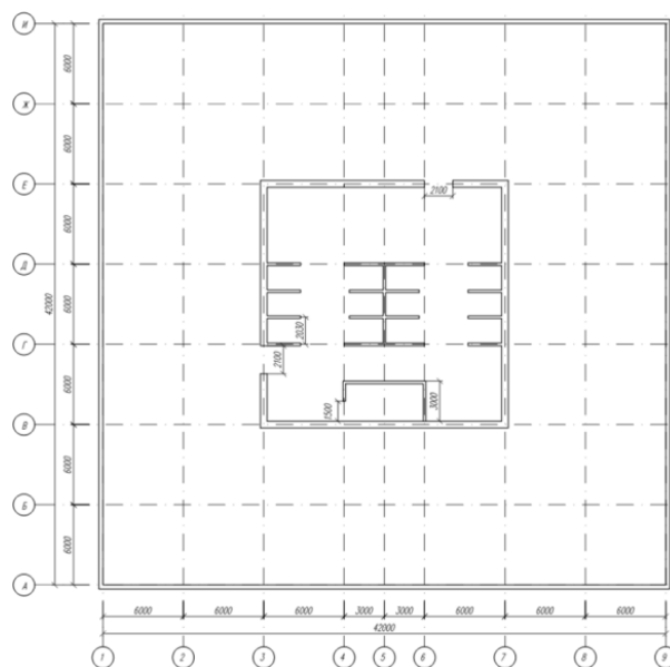
Рис. План типового этажа
