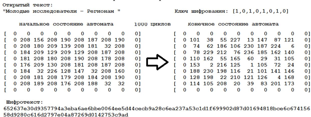
Рис. 2. Пример построения шифра с использованием клеточного автомата
