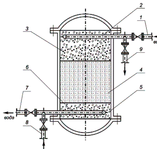
Рис. 1. Электрохимический фильтр:
