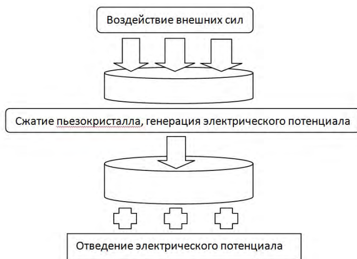
Рис. Принцип работы пьезоэлементов
