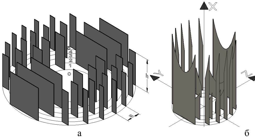
Рис. 1. Пример конструкций фазоинверторных зон из плоскопараллельных металлических пластин при: а) фокусировке на бесконечность (плоский волновой фронт на входе устройства); б) фокусировке в точку
