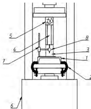
Рис. 2. Схема установки: 1 – швеллер; 2 – трубка; 3 – опора под образцом; 4 – опытный образец – балка; 5 – брус 100x100 мм; 6 – гидравлический пресс П-50; 7 – штатив; 8 – микрометр часового типа
