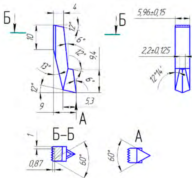
Рис. 3. Твердосплавная вставка
