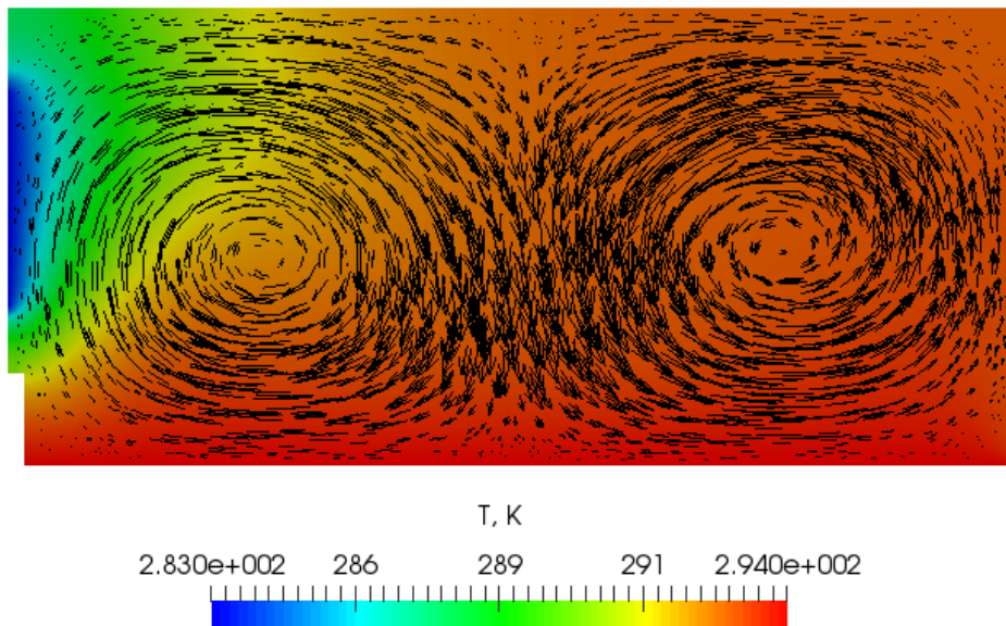
Рис. 2. Температурное поле и движение потока воздуха в комнате при использовании в качестве источника обогрева теплого пола
