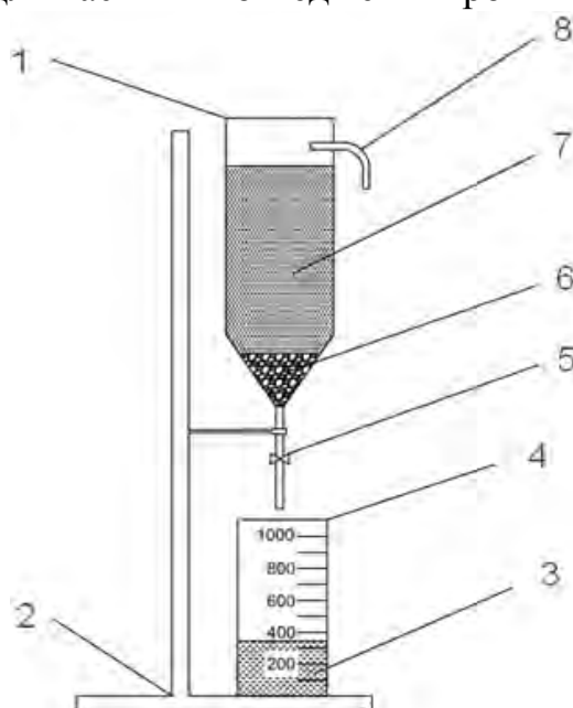
Рис. 1. Схема установки: 1 – фильтрационная емкость; 2 – штатив; 3 – очищенная вода; 4 – емкость для очищенной воды; 5 – регулировочный кран; 6 – поддерживающий слой; 7 – загрузка; 8 – переливная трубка
