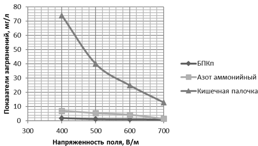
Рис. 2. Влияние напряженности электрического поля на изменения показателей очистки
