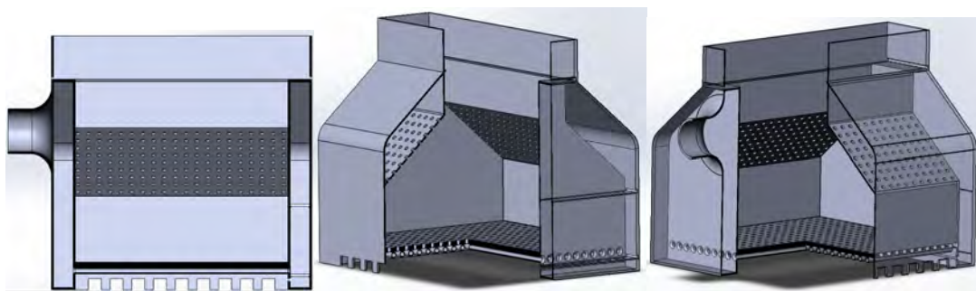
Рис. Фрагменты модели конструкции печи на обратной тяге
