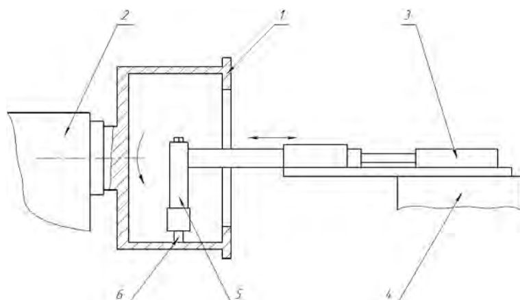
Рис. Установка для исследования износостойкости:
