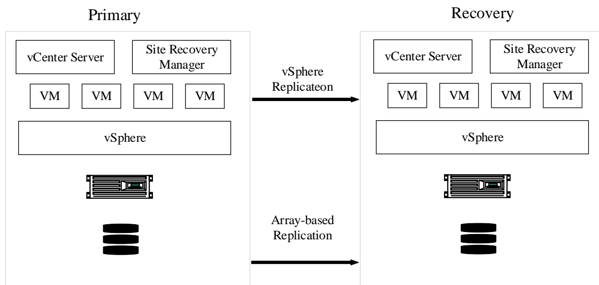
Рис. Платформа репликации
