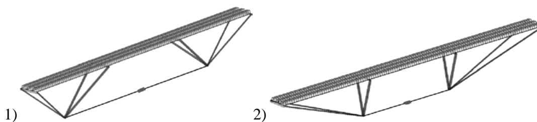
Рис. 1. Варианты шпренгеля
