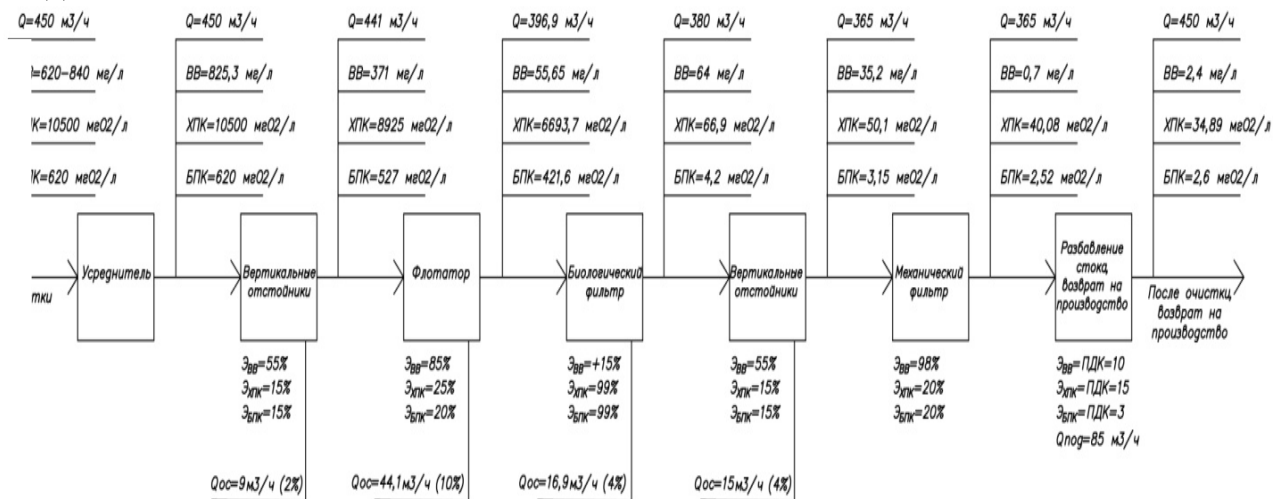
Рис. Балансовая схема очистки стока после модернизации
