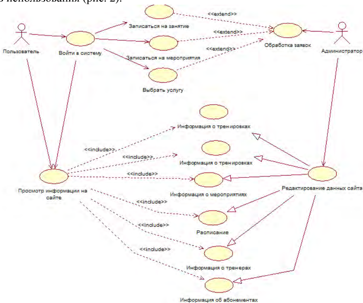
Рис. 2. Диаграмма вариантов использования
