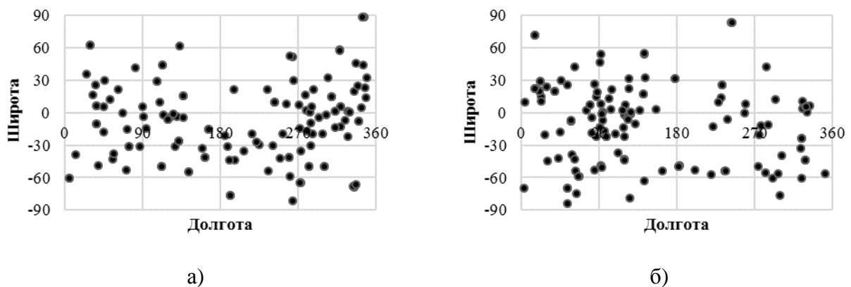
Рис. Распределение комет по долготе и широте афелия для интервалов афелийных расстояний Q : а) 100–400 а.е., б) 400–1000 а.е.
