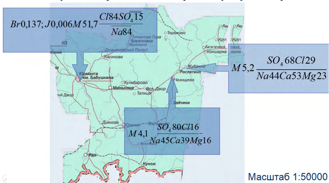
Рис. Состав минеральных вод, вскрытых разведочно-эксплуатационными скважинами на территории Бабушкинского района
