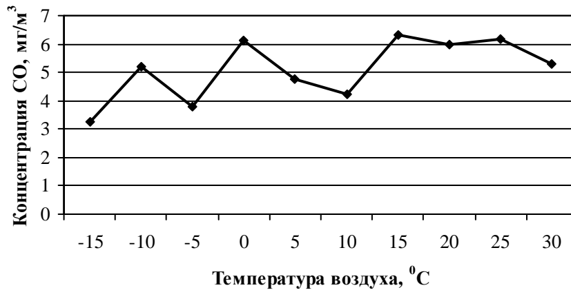
Рис. 1. Зависимость концентрации угарного газа от скорости ветра и температуры воздуха
