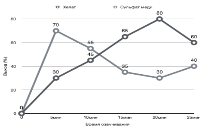
Рис. 1. Выход продукта (глицинат) и остаточное содержание \text{CuSO}_4 (%)
