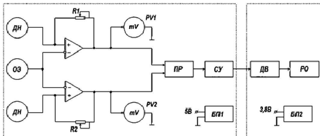
Рис. Функциональная схема разрабатываемого устройства: ДН – датчики напряжения (электроды); ОЭ – общий электрод; U1, U2 – усилители биопотенциалов с регулируемым коэффициентом усиления; ПР – аналого-цифровой преобразователь импульсов; PV1, PV2 – цифровые милливольтметры; ДВ – шаговый двигатель; БП1 – блок питания системы управления; БП2 – блок питания двигателя; СУ – система управления двигателем; РО – рабочий орган (искусственная кисть протеза)
