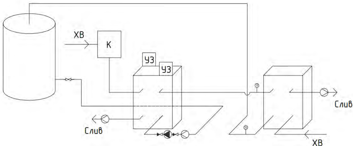
Рис. Установка по исследованию процессов теплопереноса в пластинчатых теплообменниках при участии ультразвука
