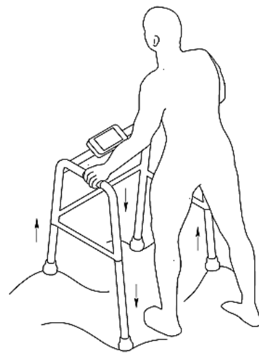
Рис. 2. Передвижение по неровной поверхности
